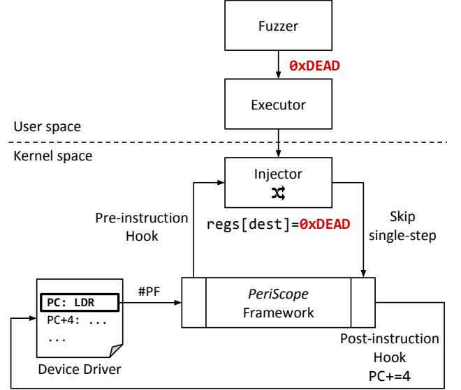
Fig. 3. PERIFUZZ overview
